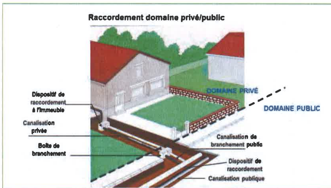
Figure 1. Description schématique d'un branchement
